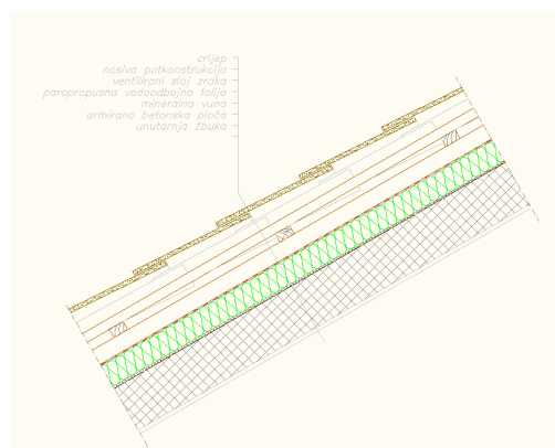
Slika 6. Izolirani krov
