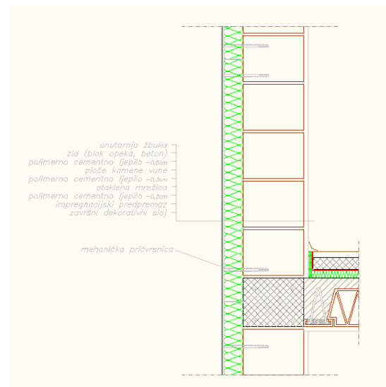
Slika 4. Izolirani zid
